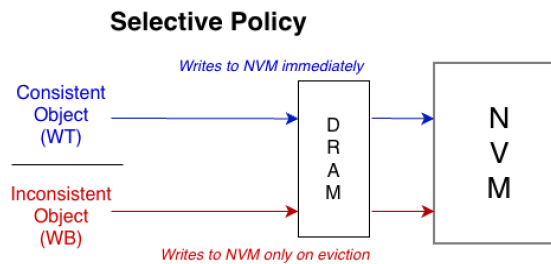
Σχήμα 4.4: Selective Policy
