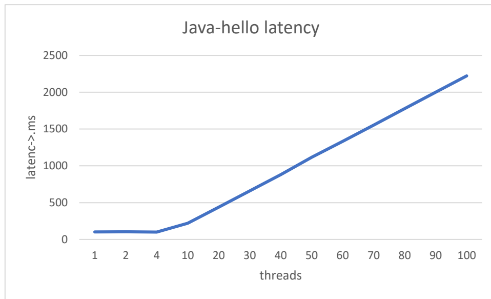
Σχήμα 4.1 Χρόνος εκτέλεσης του προγράμματος Java-hello για 1-100 νήματα
