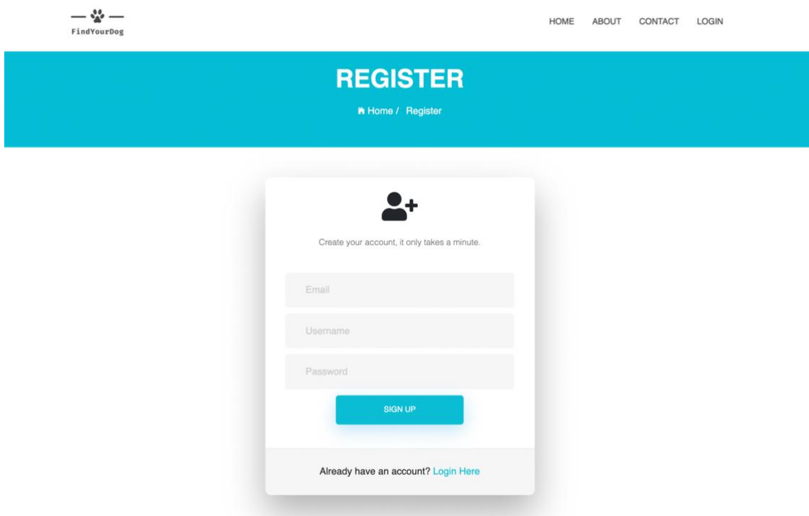
Σχήμα 6.21 Δημιουργία λογαριασμού
