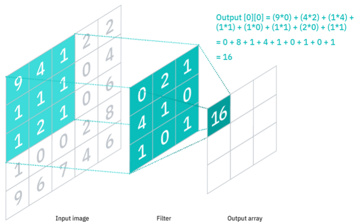
Σχήμα 4.10 Παράδειγμα Συνέλιξης
