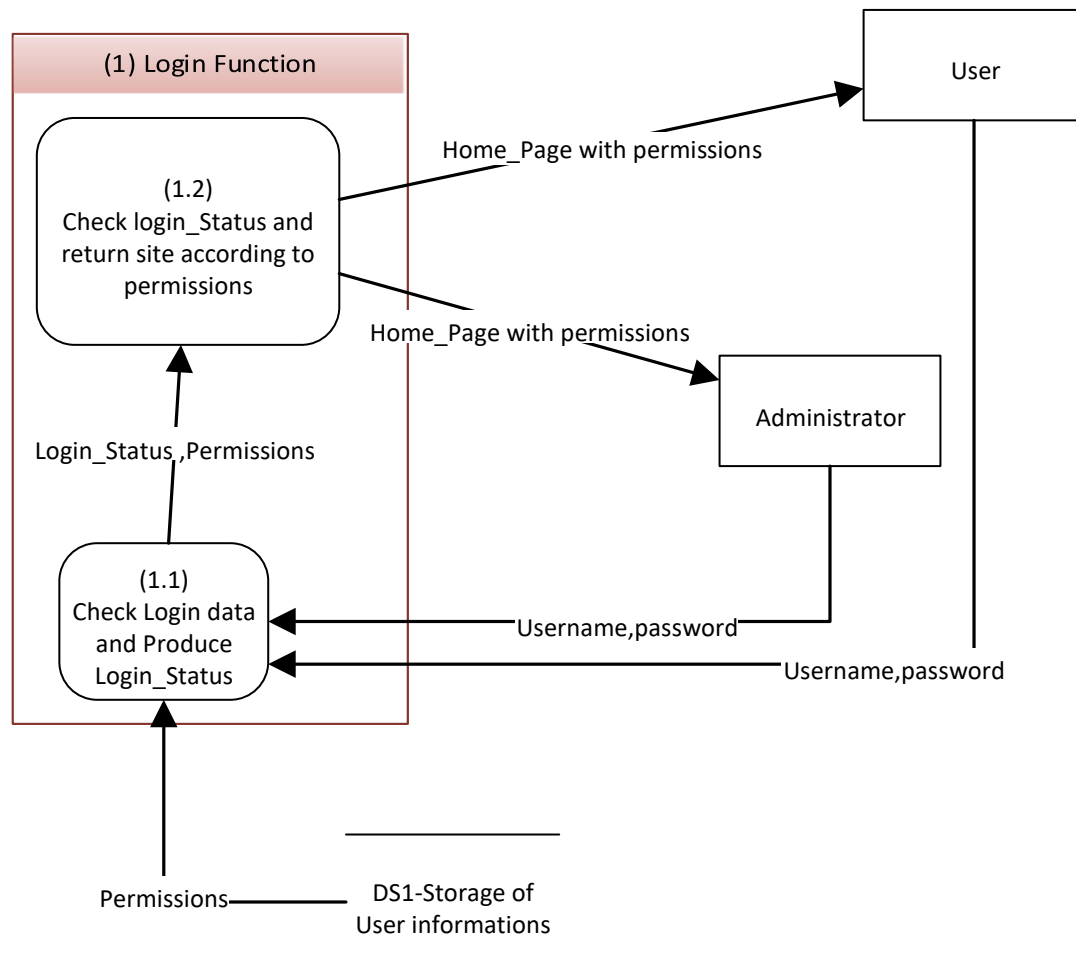
Σχήμα 3.3 Διάγραμμα Ροής Δεδομένων για την διαδικασία εισόδου του χρήστη στην εφαρμογή
