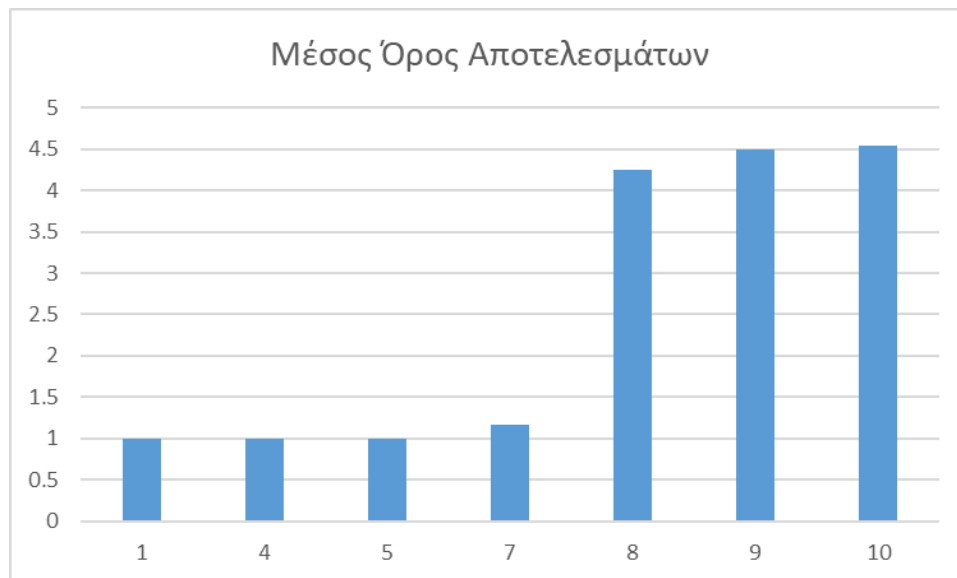
Σχήμα 7.1 Παρουσίαση του μέσου όρου των αποτελεσμάτων από τις ερωτήσεις πολλαπλής επιλογής.
