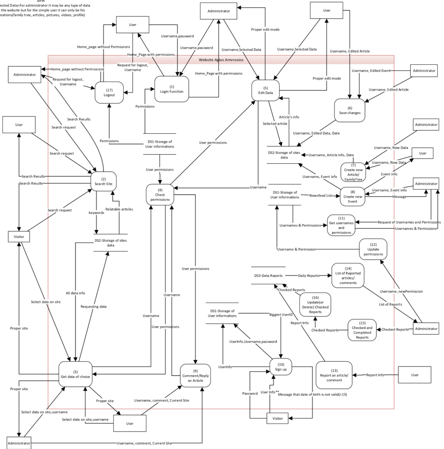
Σχήμα 3.2 Γενικό Διάγραμμα Ροής Δεδομένων της εφαρμογής
