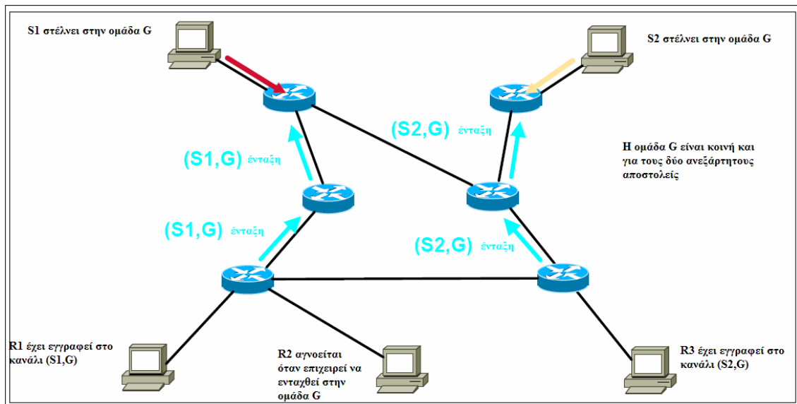
Σχήμα 3.9 – Εγγραφή R1 και R3 στην ίδια ομάδα
