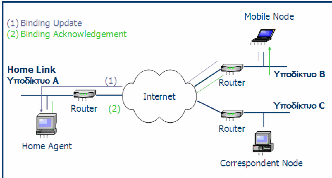
Σχήμα 1.3 – Διαδικασία εγγραφής του Home Agent
