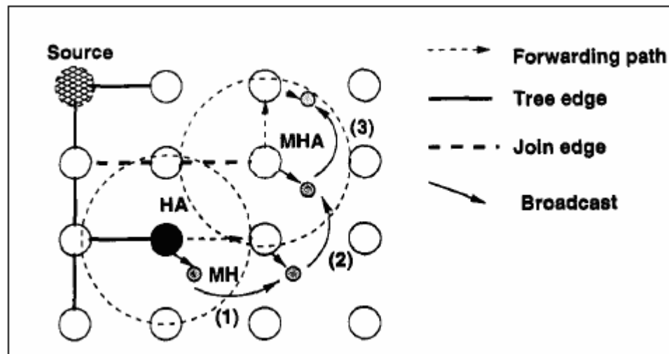
Σχήμα 3.2 – Μετακίνηση του κινητού χρήστη
