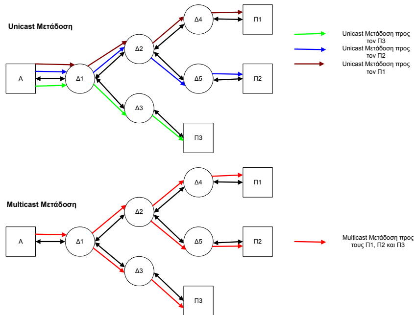
Σχήμα 1.2 – Μετάδοση multicast και unicast
