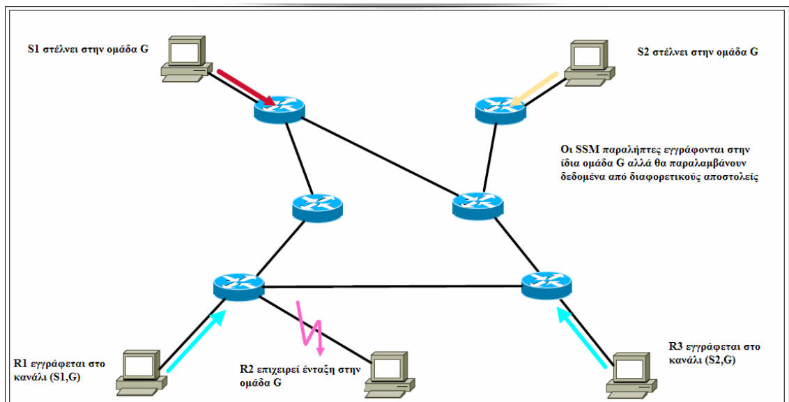
Σχήμα 3.8 - Εγγραφή R1 και R3 στην ομάδα
