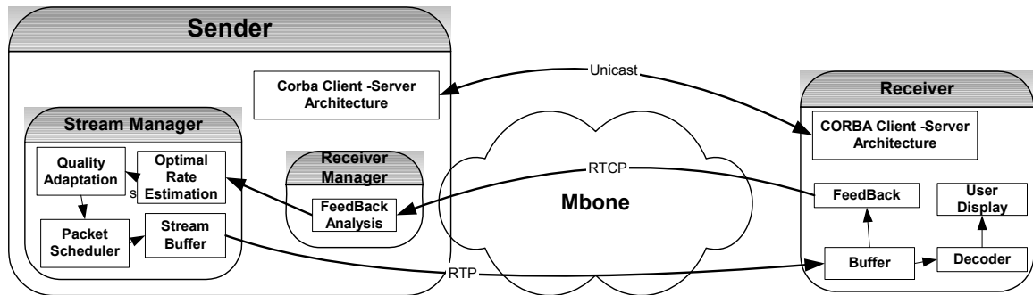
Σχήμα 2.9 – Λειτουργία του προτεινόμενου μηχανισμού
