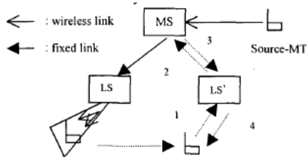
Σχήμα 2.2 – Handoff του παραλήπτη
