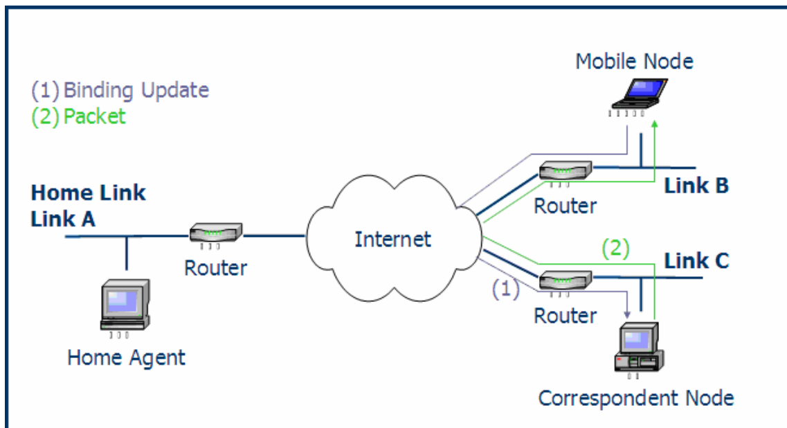
Σχήμα 1.5 – Διαδικασία Binding Update
