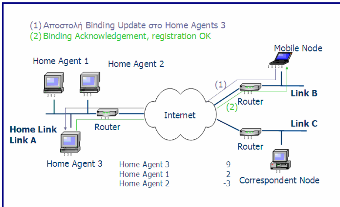
Σχήμα 1.7 – Επιτυχής εγγραφή του Home Agent 3
