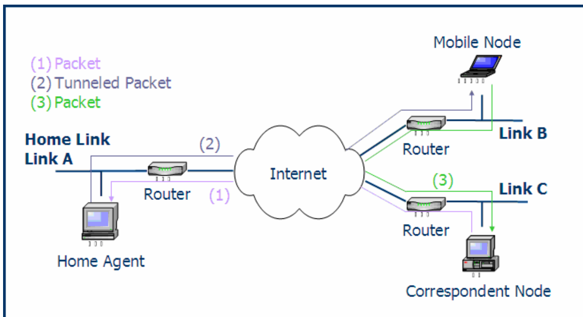
Σχήμα 1.4 – Δρομολόγηση πακέτου
