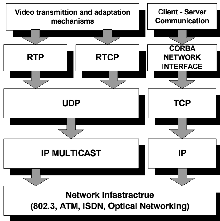
Σχήμα 2.7 – Στοιβά πρωτοκόλλων
