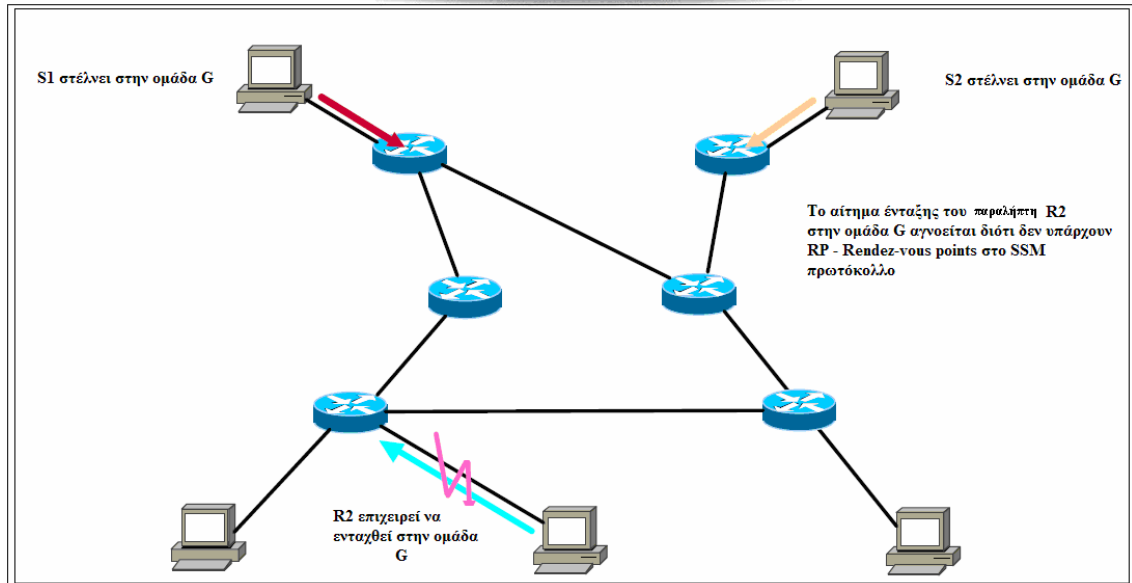
Σχήμα 3.7 – Απόρριψη παραλήπτη R2 να ενταχθεί σε κανάλι
