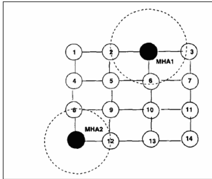
Σχήμα 3.1 – Τοπολογία για το RBMoM
