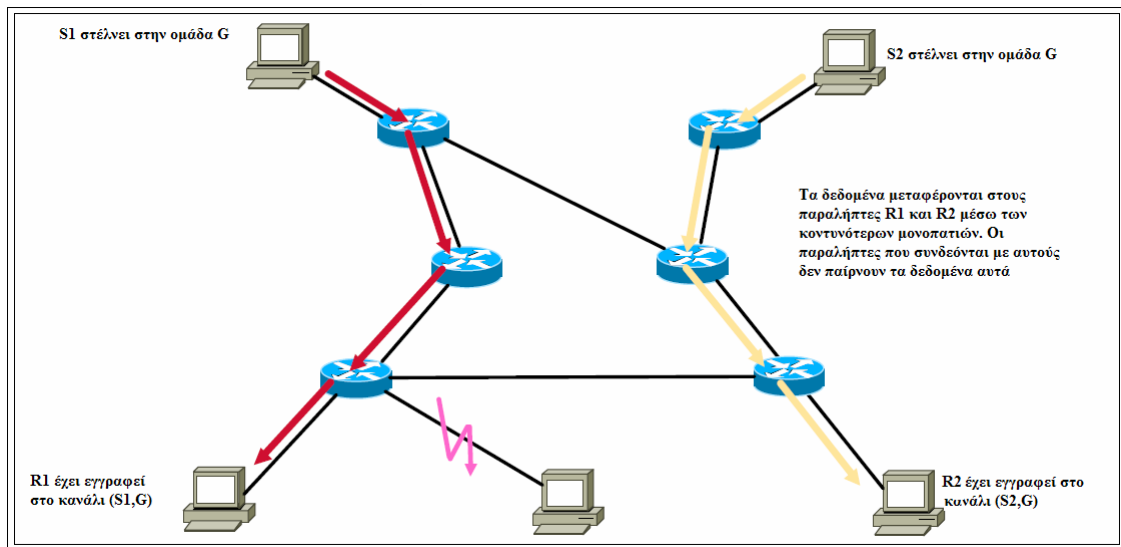
Σχήμα 3.10 – Μεταφορά δεδομένων
