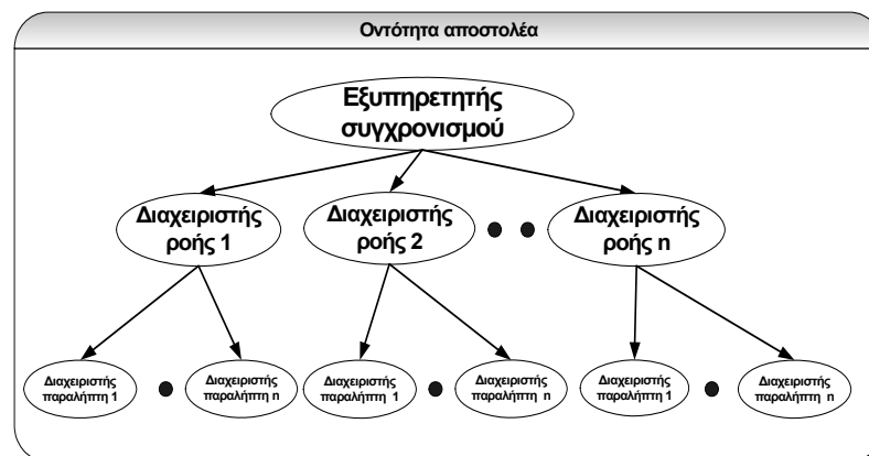
Σχήμα 2.8 – Αρχιτεκτονική αποστολέα
