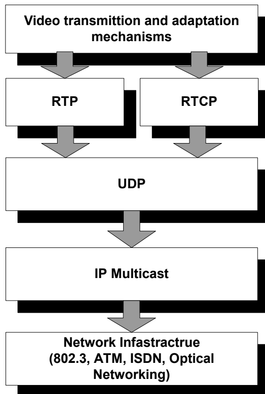
Σχήμα 2.6 – Στοίβα πρωτοκόλλων
