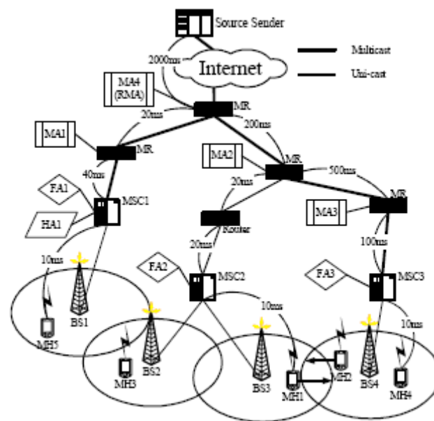
Σχήμα 2.4 – Αναπαράσταση πρωτοκόλλου
